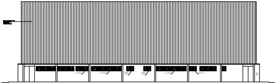
GINÁSIO - ELEVÇÃO 01 ESC. 1:50
