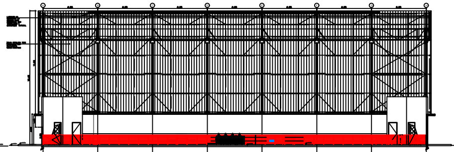
GINÁSIO - CORTE B ESC. 1:50
