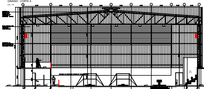
GINÁSIO - CORTE A (APENAS PARA GINÁSTICA ARTÍSTICA) ESC. 1:50
